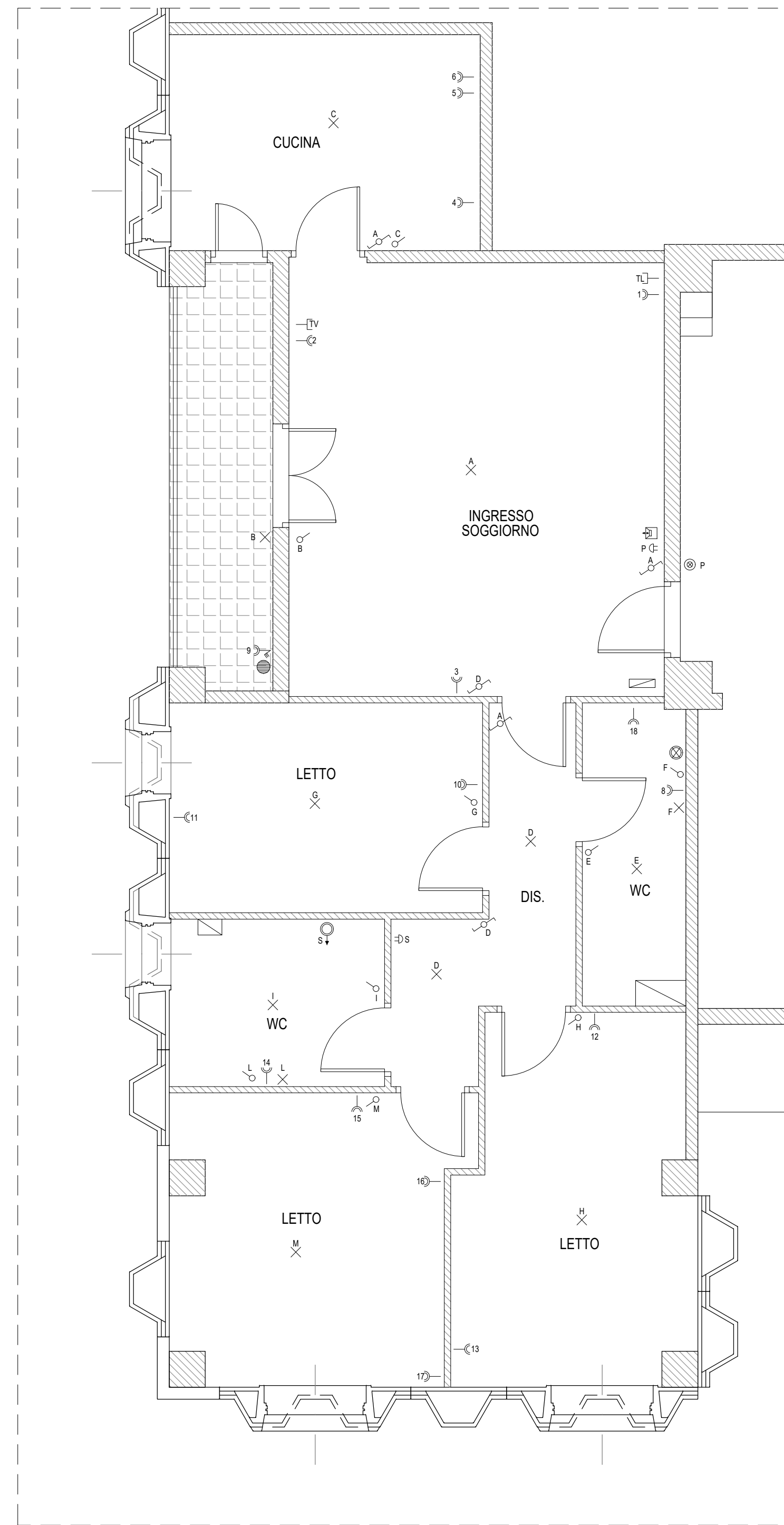
PIANTA ALLOGGIO TIPO 90 mq SCALA 1:50
