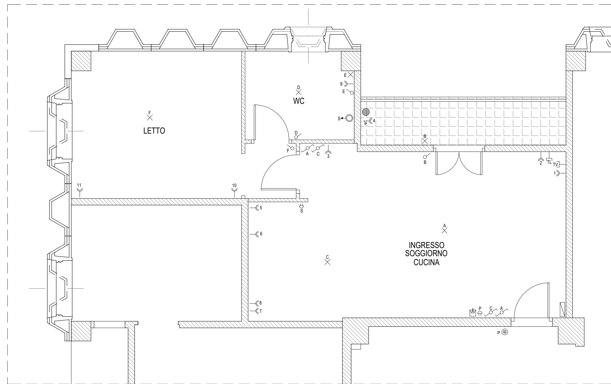
PIANTA ALLOGGIO TIPO 46 mq SCALA 1:50
