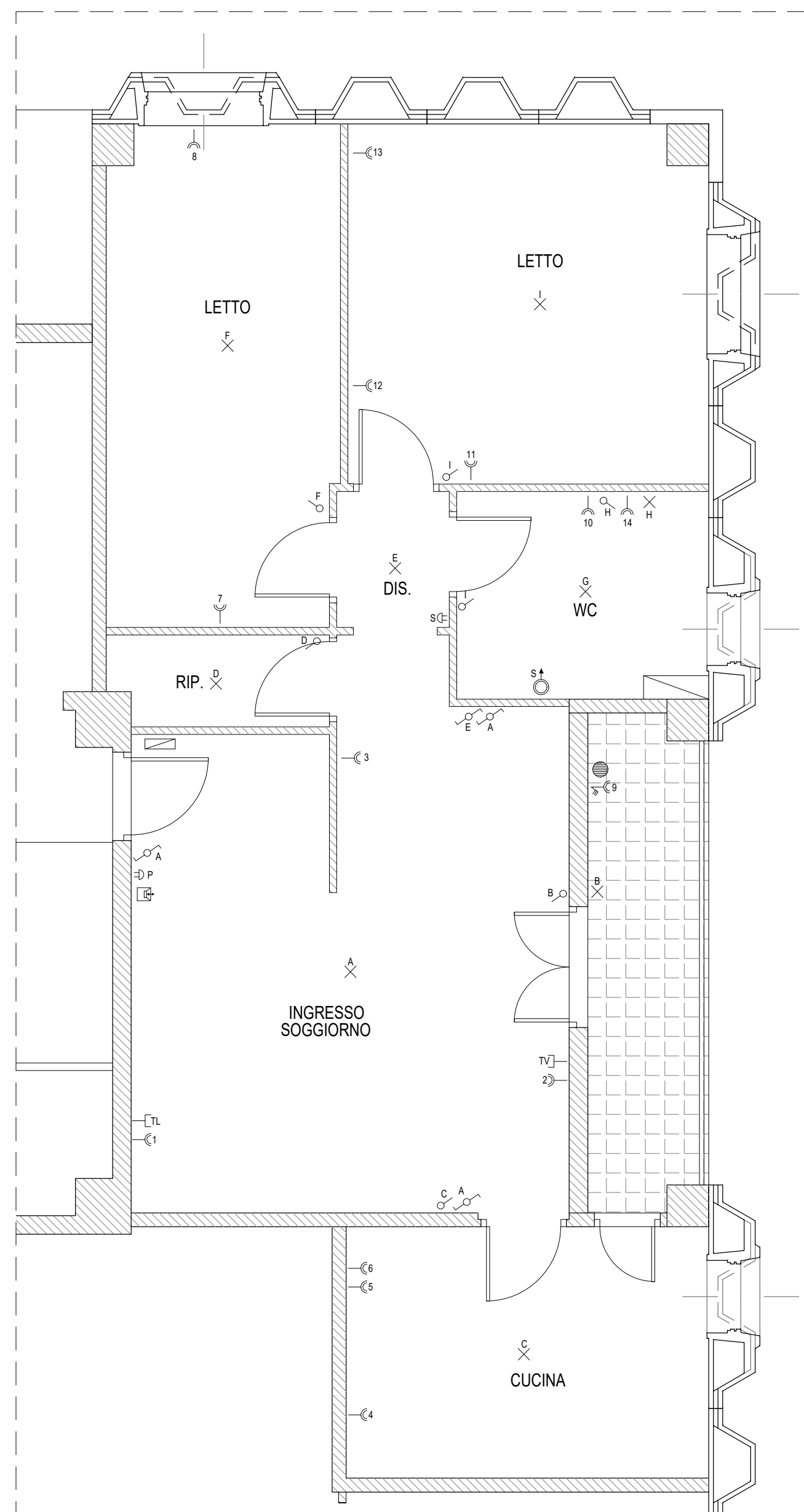
PIANTA ALLOGGIO TIPO 75 mq SCALA 1:50
