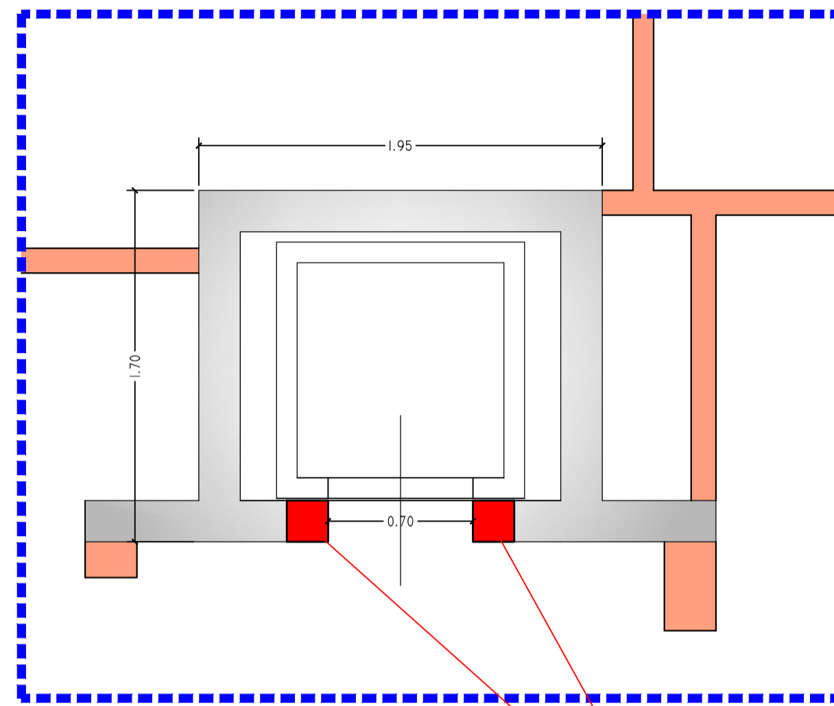
IMPIANTO ASCENSORE STATO DI FATTO
