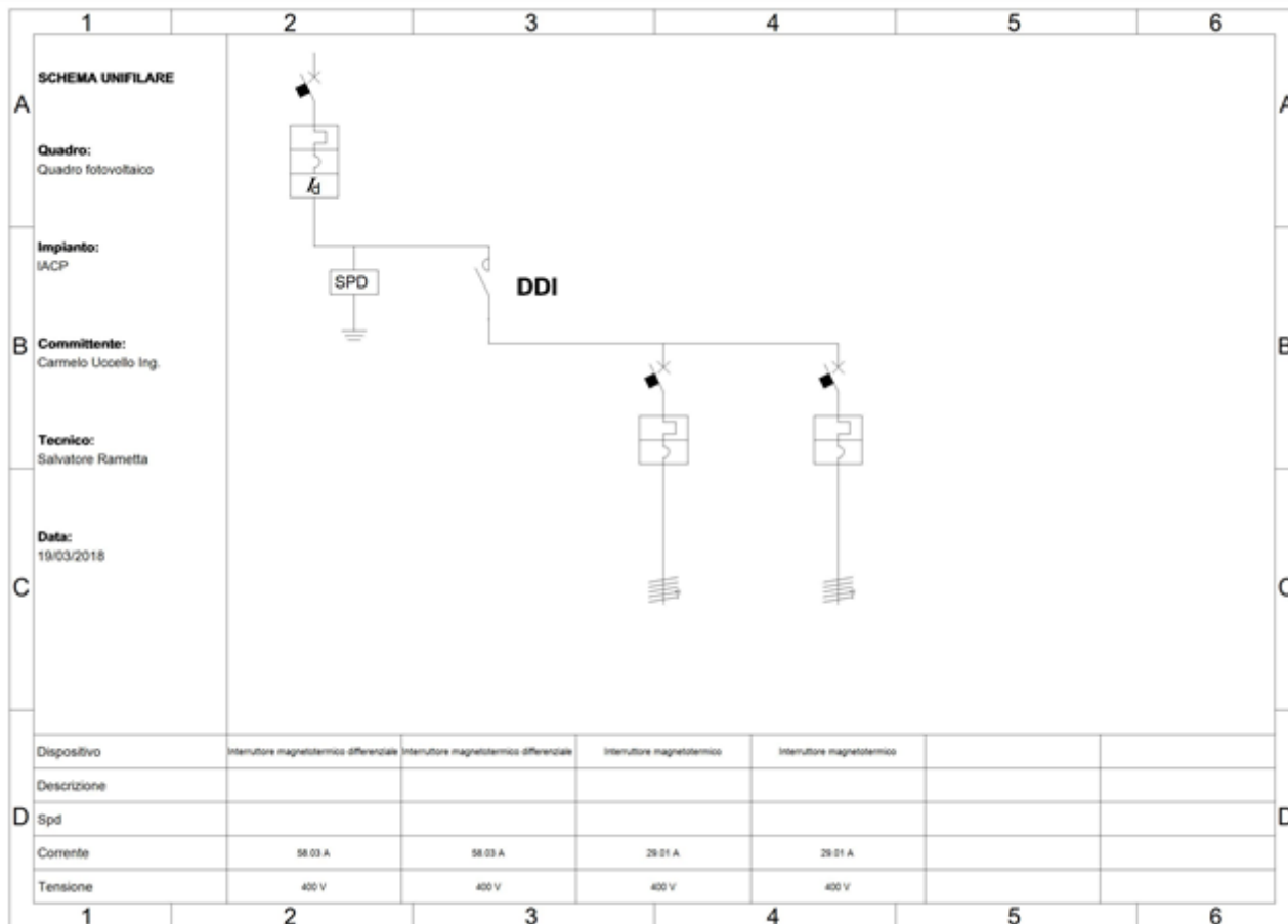
Fig. 6: Schema unifilare quadro "Quadro fotovoltaico"
