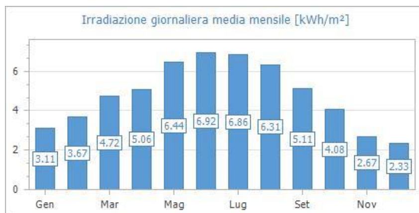
Fig. 1: Irradiazione giornaliera media mensile sul piano orizzontale [kWh/m 2 ]- Fonte dati: UNI 10349:2016 - Stazione di rilevazione: Siracusa
