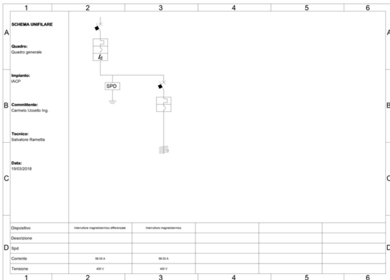
Fig. 5: Schema unifilare quadro "Quadro generale"
