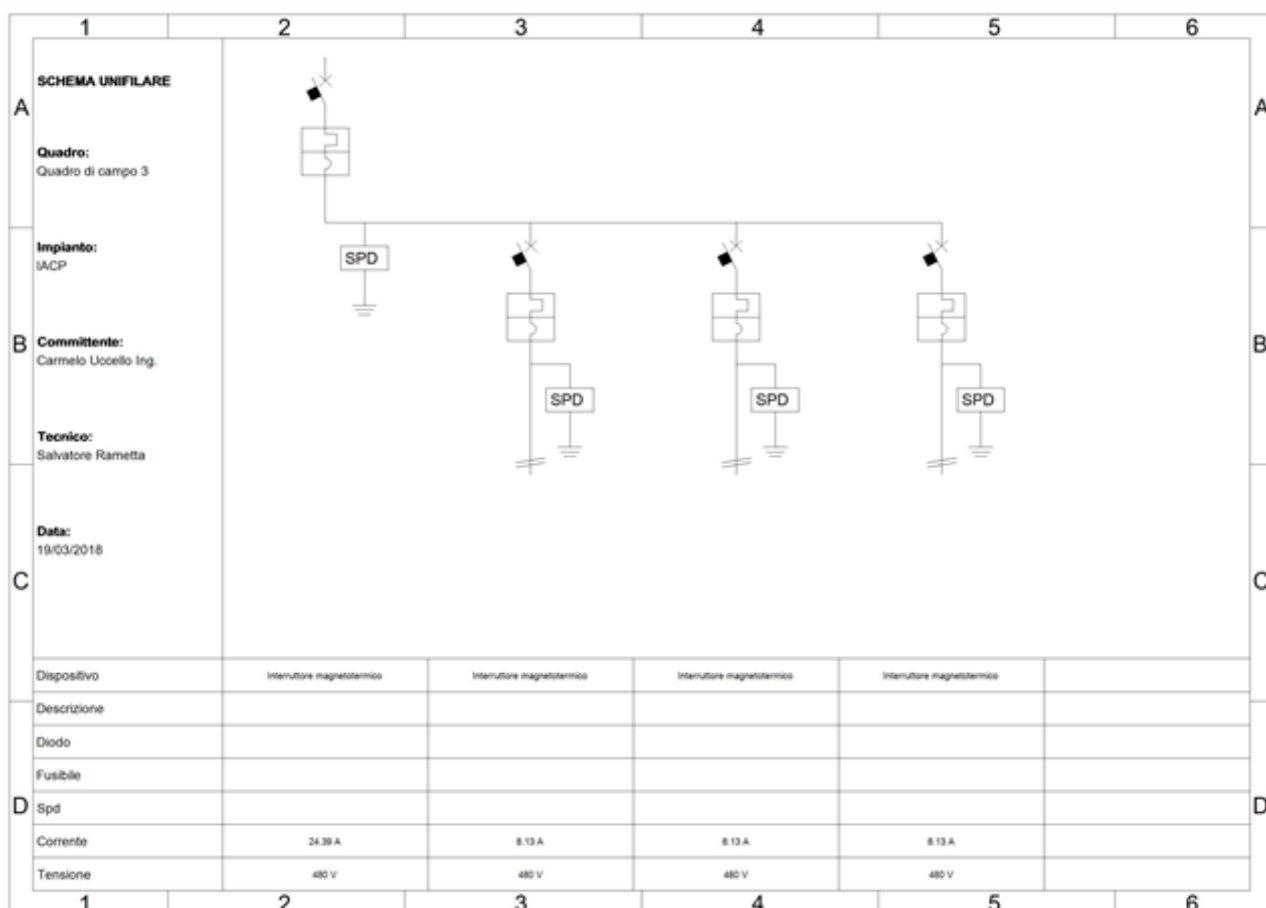
Fig. 9: Schema unifilare quadro "Quadro di campo 3"
