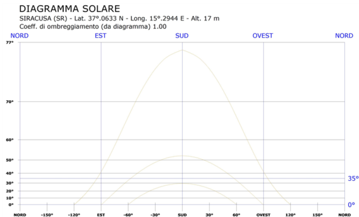
Fig. 2: Diagramma solare
